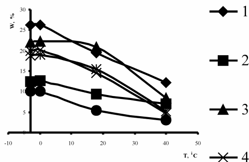
Рис. 4. Вплив температури на поглинаючу спроможність матеріалів по відношенню до дизпалива:
